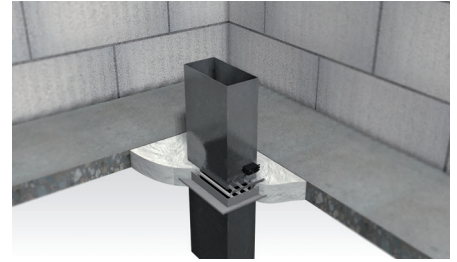
Horizontaal/verticaal – luchtklep
