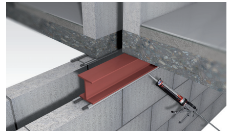
Horizontale bewegingsvoeg
