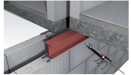
Horizontale bewegingsvoeg
